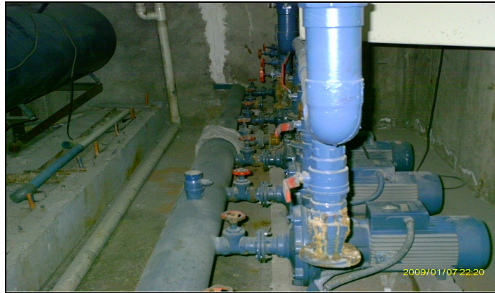
BOMBAS Y MANIFOLD DEL CIRCUITO DE BAJA
